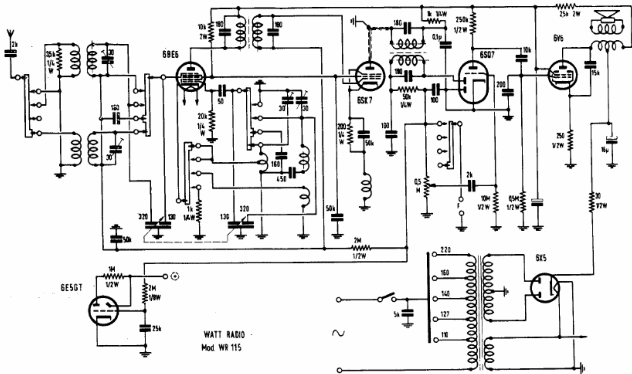
Schema elettrico del radioricevitore WATT RADIO, mod. WR 115
